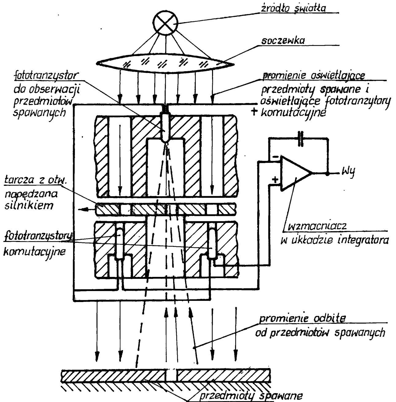
Rys.1 Schematyczne przedstawienie zasady działania czujnika.
