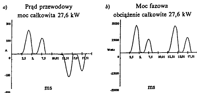
Rys. 4. Przykładowe wyniki pomiarów układów z użyciem falowników wykonane na stacji prób OBR MiR REDOR
